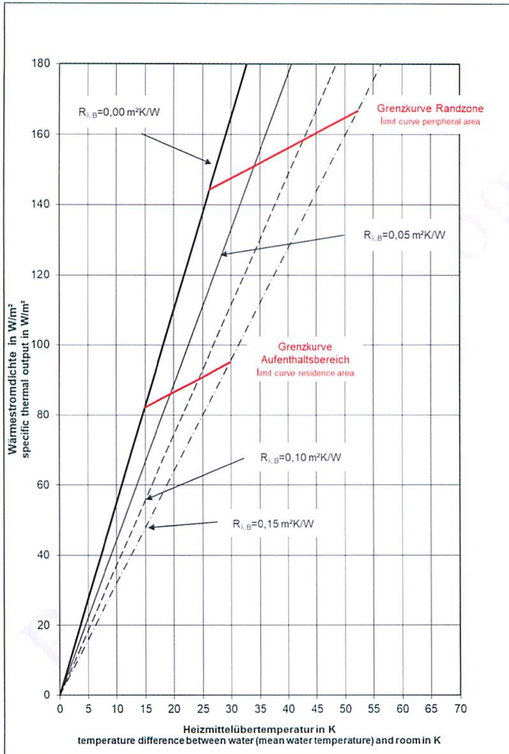
Abbildung 5: Leistungskennlinien Fußbodenheizungssystem
