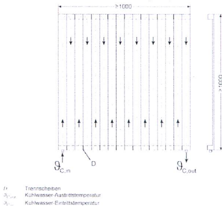
Abbildung 2: obere und untere Kühlplatte nach EN 1264 Teil 2 Abschnitt 9
