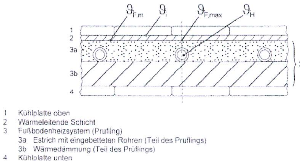
Abbildung 1: Prüfstand nach EN 1264 Teil 2 Abschnitt 9
