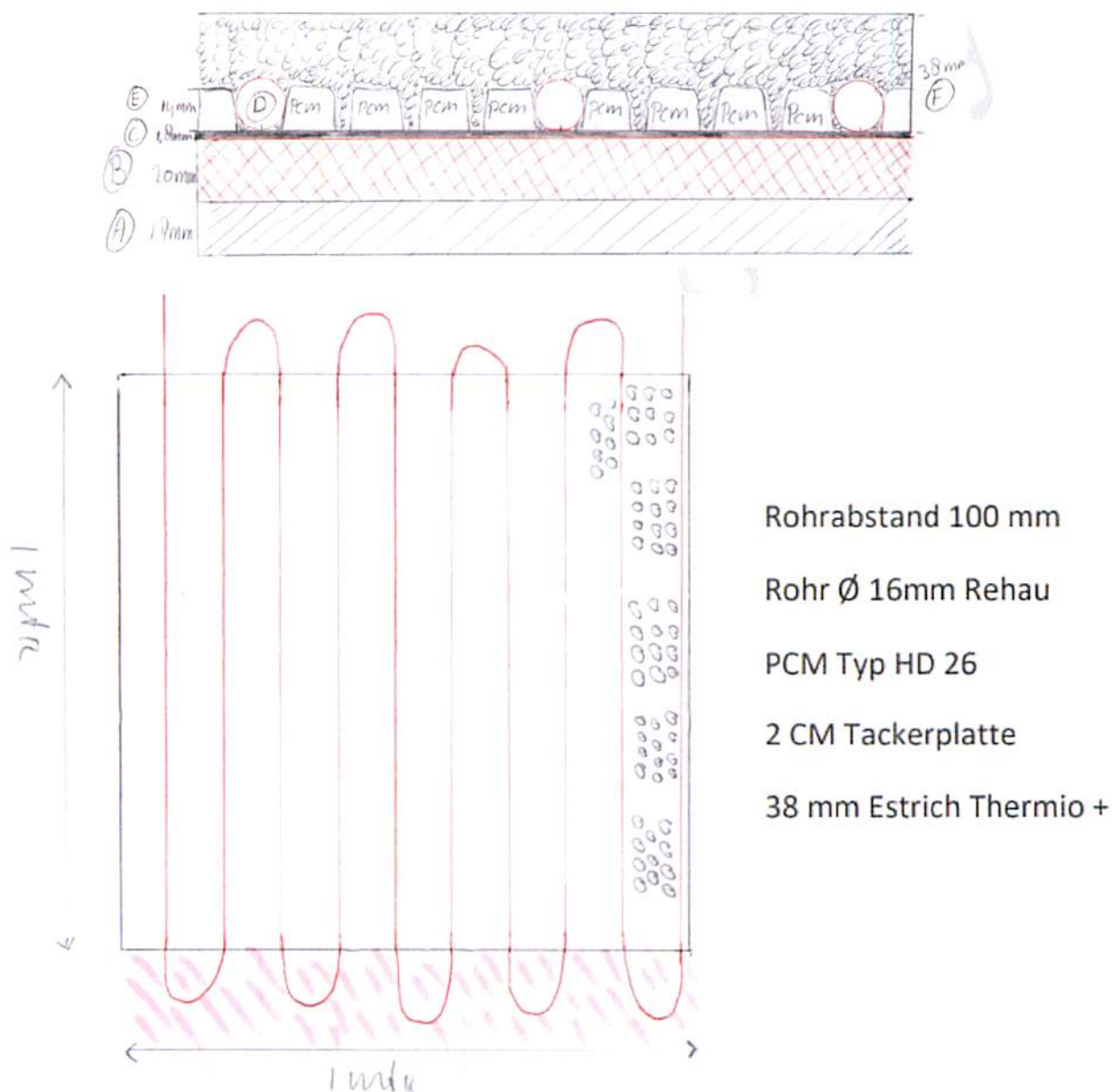
Abbildung A3: Systemaufbau
