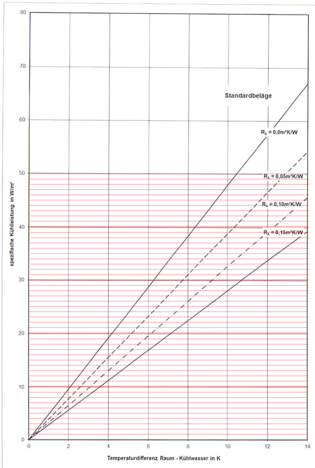
Abbildung 1: Kühlleistung in Abhängigkeit der Untertemperatur für Rohrabstand RA 100mm figure 1: cooling output in dependence of the temperature distance room - water for pipe distance RA 100 mm
